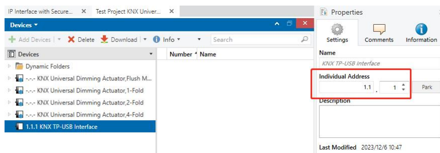
图 4.2 ETS 属性界面-实际物理
